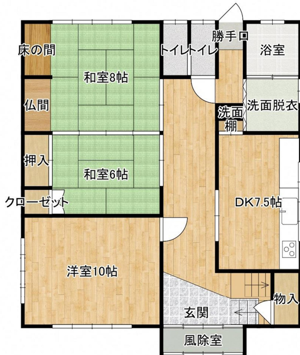
1 階
